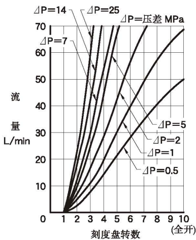
开度-流量特性
